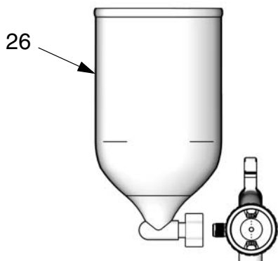
Vue en détail d'un pistolet alimenté par gravité avec réservoir latéral
